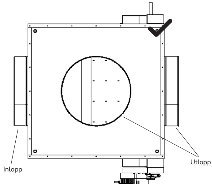
Spjällställdon placerat på höger sida (riktat nedåt)
